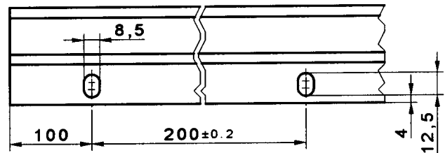
Lochung der Lasche Fig. 3 und Fig. 4
